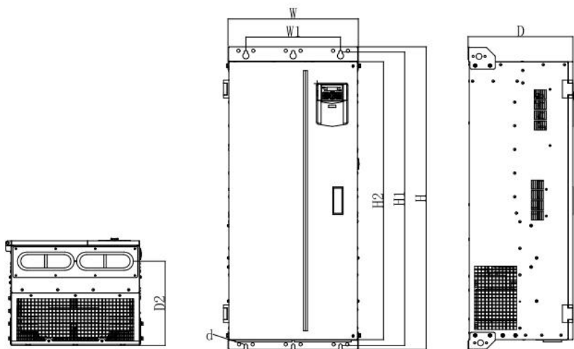
(d) EM730-185-3~EM730-220-3 变频器外形
