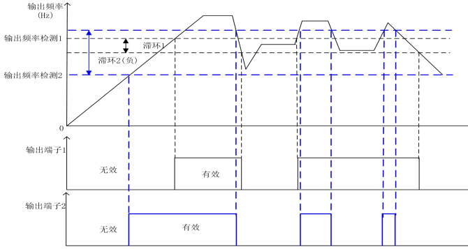
图 7- 37 FDT 检测示意图
