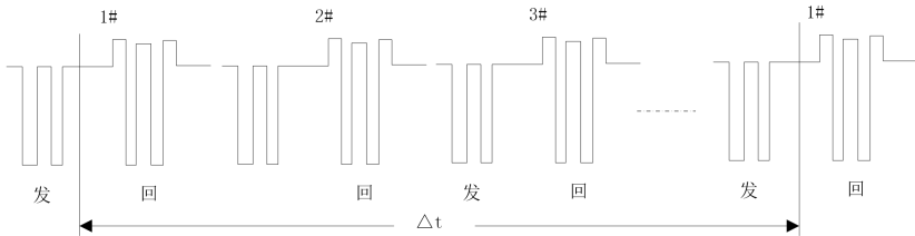
图 4- 24485 网络链路数据示意图
