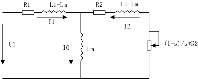
图 8-18 三相异步电动机等效电路
