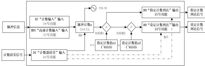
图 7- 42 计数功能框图描述
