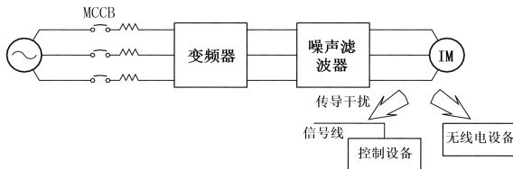
图 3-7 输出侧安装噪声滤波器
