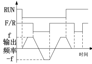
(a) F00.03=0 两线控制接线示意图 (b) F04.19=0, F00.03=0 运行正/反转逻辑
