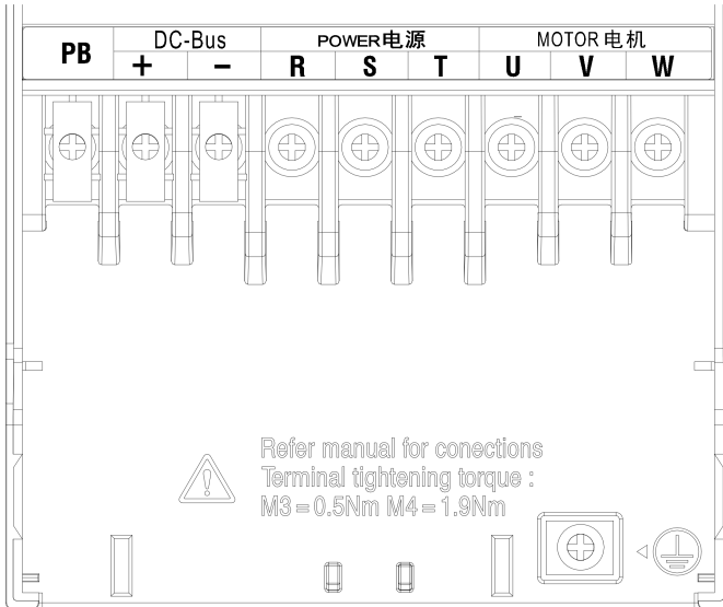
(c) EM730-5R5-3B~EM730-022-3B 端子示意图, 接地位置略有差异
