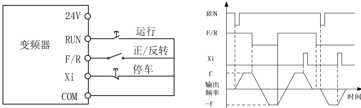
(c) F00.03=3 三线控制接线示意图 (d) F04.19=0, F00.03=3 正/反转运行逻辑
