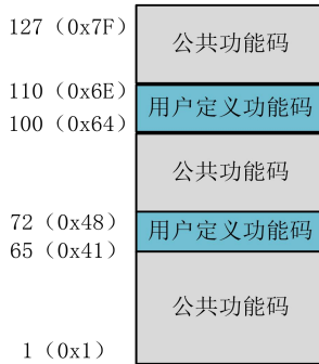
图 12- 21 MODBUS 功能码分类
