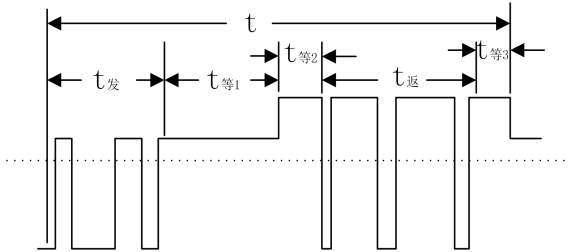
图 4- 23 完整数据帧时序解析图
