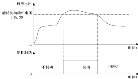
图 7- 39 能耗制动示意图
