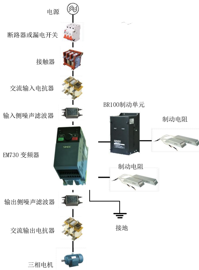
图 3- 1 变频器与外围设备的连接图
