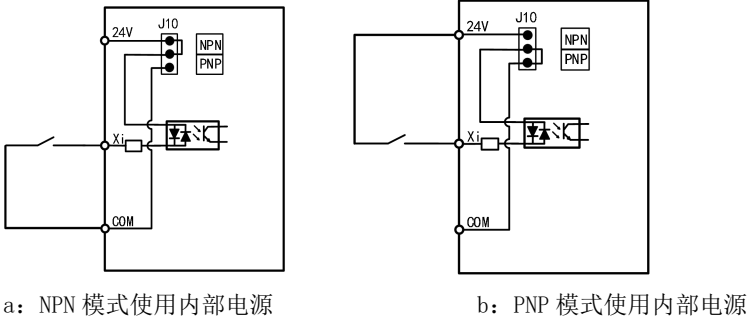
a: NPN 模式使用内部电源
