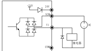
b: 使用外部电源 PNP
