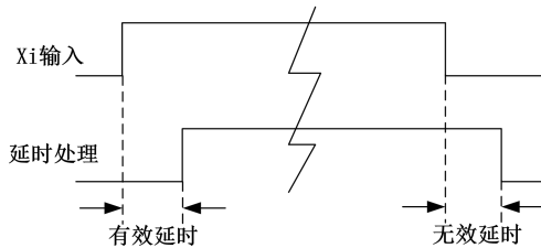
图 7- 14 端子延时采样示意图
