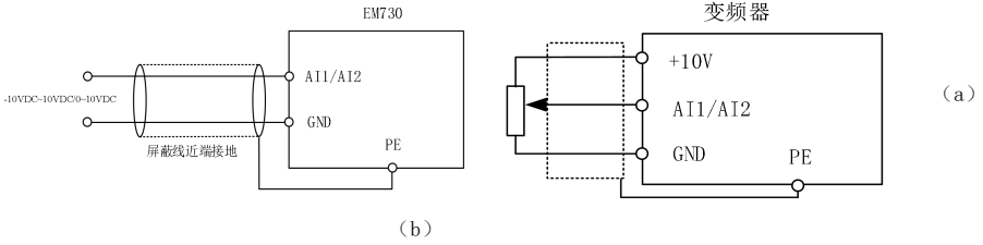
图 3- 12 AI1、AI2 端子配线图
