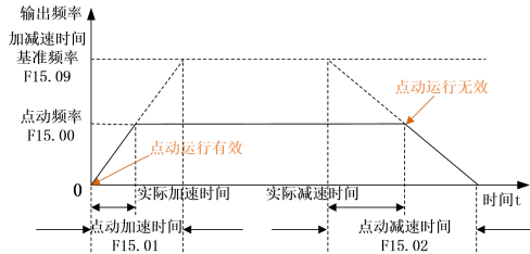
图 7- 32 点动运行示意图
