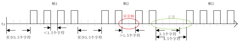
图 4- 22 数据帧正误示意图
