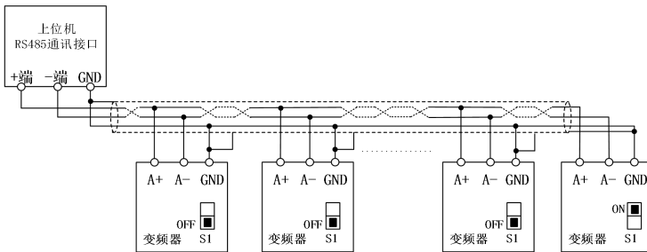
图 3- 17 多台变频器通讯端子配线
