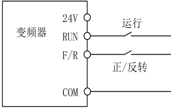
(a) F00.03=0 两线控制接线示意图
