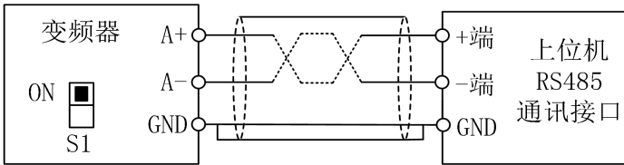
图 3- 16 单台变频器通讯端子配线
