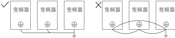
图 3- 10 接地线连接方法
