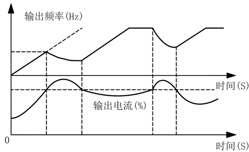
图 7- 25 电流限幅动作过程
