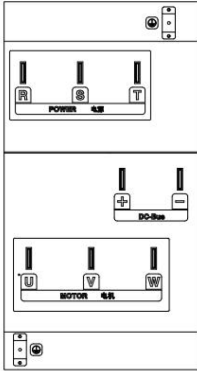
(h) EM730-280-3~EM730-450-3 端子示意图
