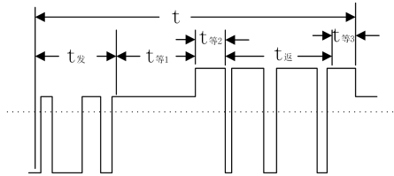
图 7- 31 完整数据帧时序解析图
