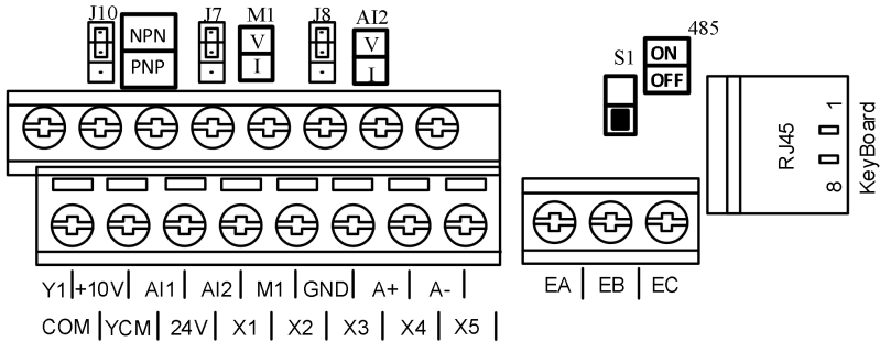
图 3-11 控制回路端子排列
