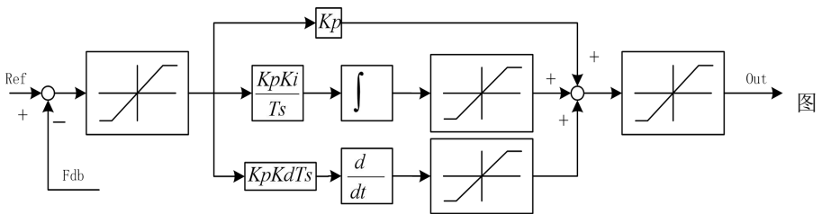
7- 27 过程 PID 框图描述
