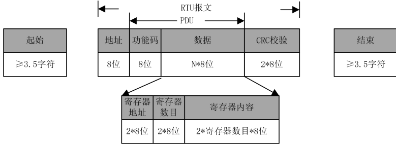
图 12- 20 RTU 模式报文帧示意图
