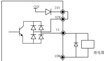
a: 使用内部电源 PNP
