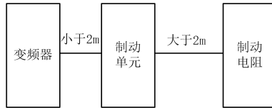
图 4- 19 导线的长度
