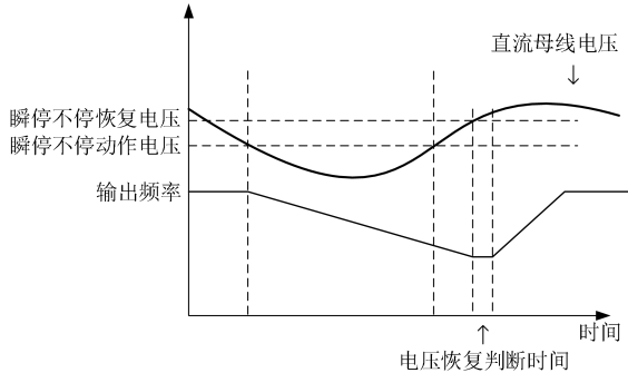
图 7- 24 瞬停不停减速功能动作示意图
