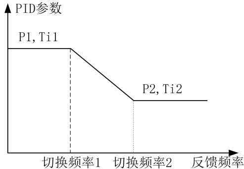
图 7- 21 PI 参数示意图
