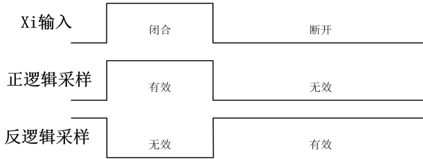
图 7- 12 端子正反逻辑采样示意图
