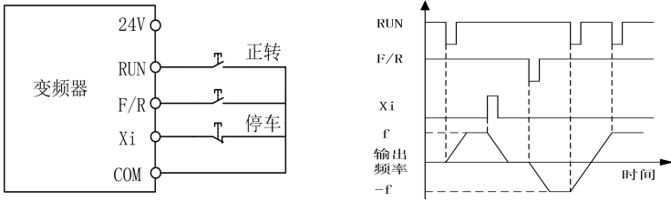
(a) F00.03=2 三线控制接线示意图 (b) F04.19=0, F00.03=2 正/反转运行逻辑
