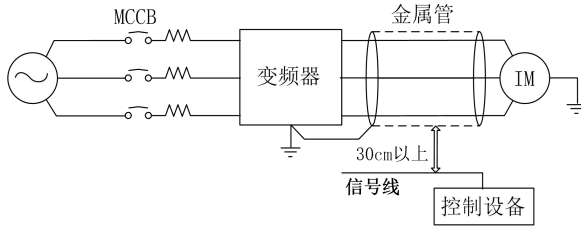
图 3- 8 感应干扰对策
