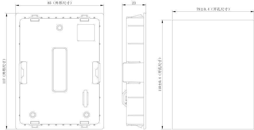
(a) 键盘托架尺寸
