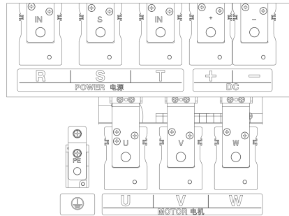
(d) 132-220kW 主回路端子
