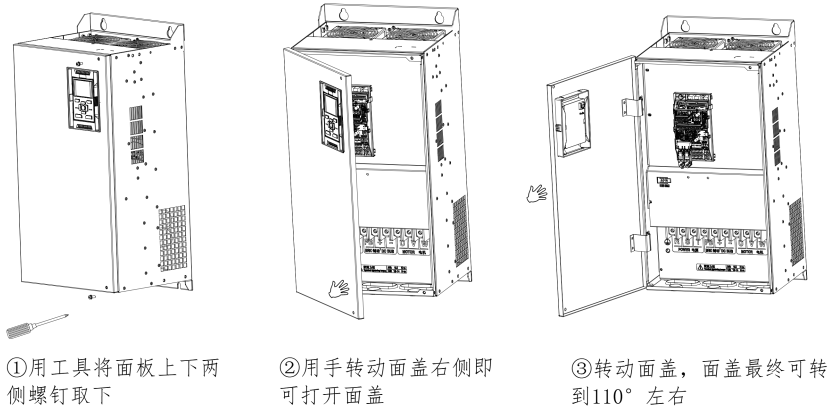
图 2- 4 030G/037P~400G/450P 面板拆卸示意图
