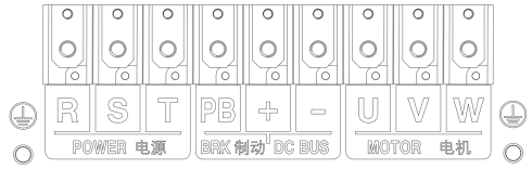
(b) 30-75kW 主回路端子 (-3 系列没有 PB 端子)
