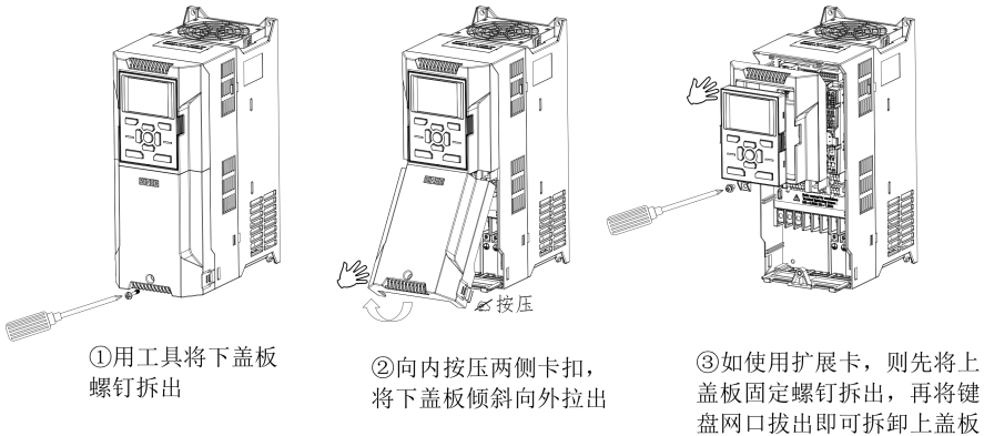
图 2- 3 0R7G/1R5P~022G/030P 面板拆卸示意图
