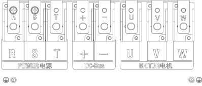
(c) 90-110kW 主回路端子
