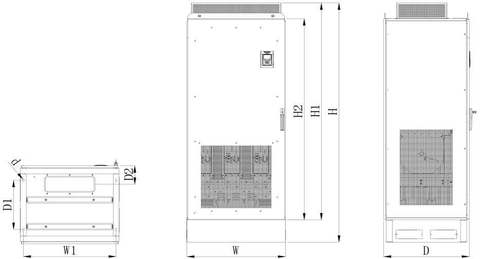
(d) 450G/500P~560G/630P 变频器外形
