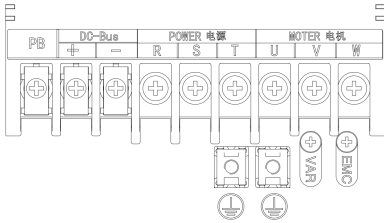
(a) 0.75-22kW 主回路端子
