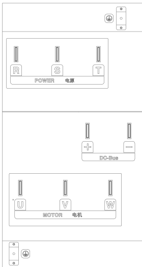
(e) 250-400kW 主功率端子
