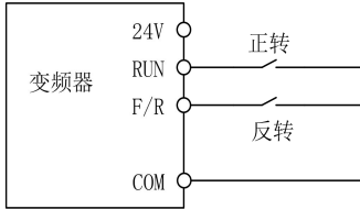
(c) F00.03=1 两线控制接线
