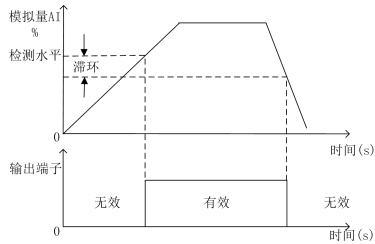
图 7- 38 ADT 检测示意图
