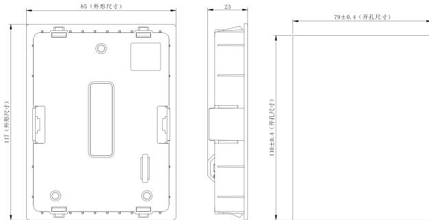
(K) EM750 外引键盘托架外形及开孔尺寸要求
