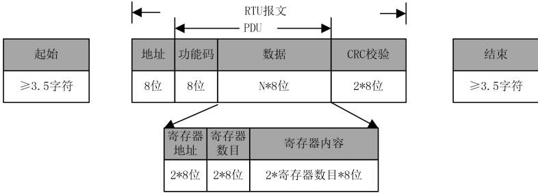
图 12- 20 RTU 模式报文帧示意图
