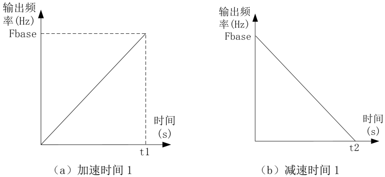
图 7- 9 加减速时间
