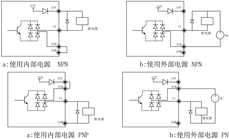
图 3-15 多功能输出端子接线方式
