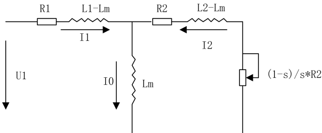
图 7- 11 异步电动机稳态等效模型
