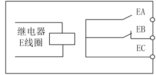
图 7- 12 继电器触点
