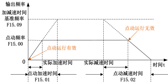
图 7- 32 点动运行示意图
