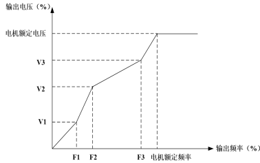
图 7-19 多点折线 V/F 曲线示意图
