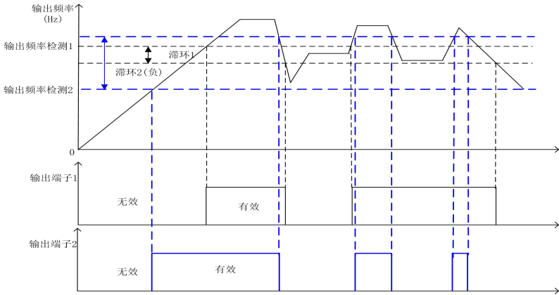
图 7- 37 FDT 检测示意图
