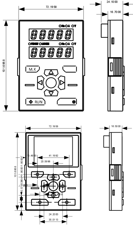
(J) EM750 外引键盘外形及尺寸
