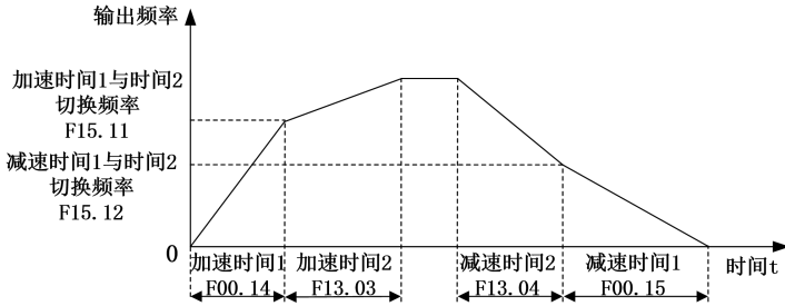
图 7-34 加减速时间自动示意图
