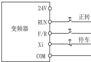
(a) F00.03=2 三线控制接线示意图
