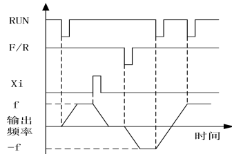
(b) F04.19=0, F00.03=2 正/反转运行逻辑
