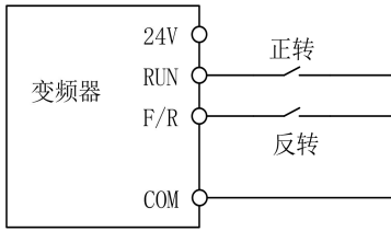
(c) F00.03=1 两线控制接线示意图 (d) F04.19=0, F00.03=1 正/反转运行逻辑
