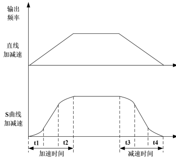
图 7-16 加减速时间控制图
