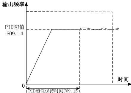
图 9- 29 PID 初值输出示意图
