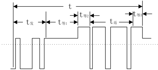
图 4- 23 完整数据帧时序解析图
