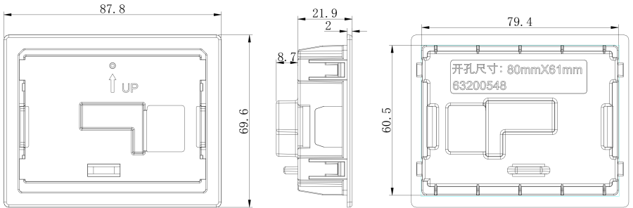
(I) EM750 键盘托架外形及开孔尺寸要求
