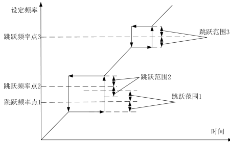
图 7- 35 跳频示意图
