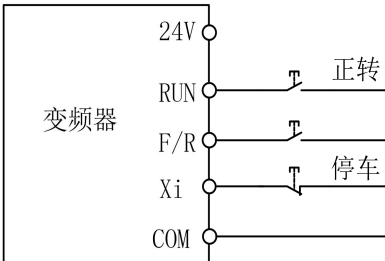
(a) F00.03=2 三线控制接线示意图
