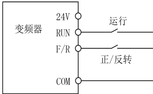
(a) F00.03=0 两线控制接线示意图 (b) F04.19=0, F00.03=0 运行正/反转逻辑
