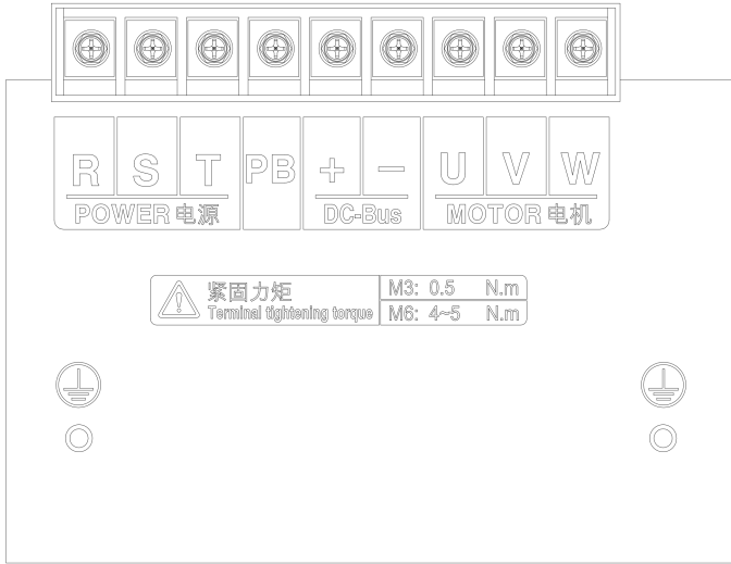
(d) EM750-030G/037P-3/3B~EM750-037G/045P-3/3B 端子示意图
