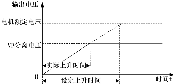
图 7- 20 VF 分离电压上升时间说明
