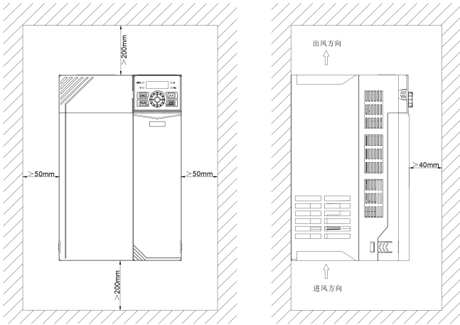
图 2- 2 变频器安装方向和空间
