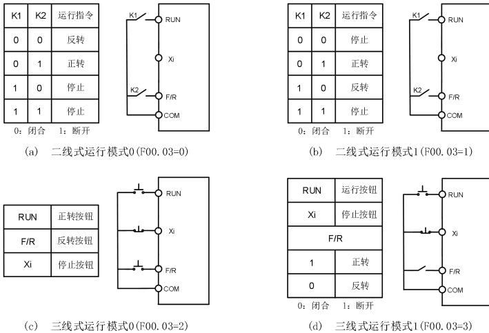
图 1- 6 端子运行方式控制逻辑图
