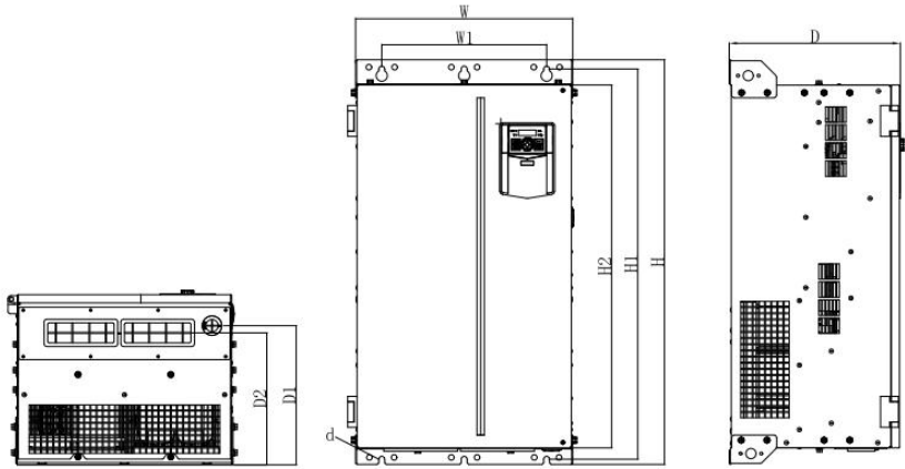
(d) EM750-185G-3~EM750-220G-3 变频器外形
