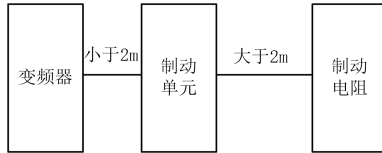
图 4- 19 导线的长度
