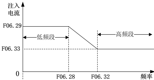
图 7- 22 高频注入图示
