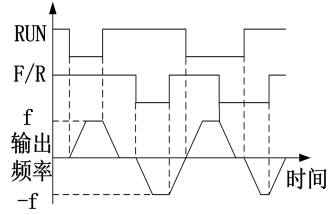
(c) F00.03=1 两线控制接线示意图 (d) F04.19=0, F00.03=1 正/反转运行逻辑
