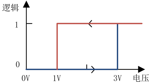
图 7- 10 模拟输入端子电压与当前逻辑状态对应关系图
