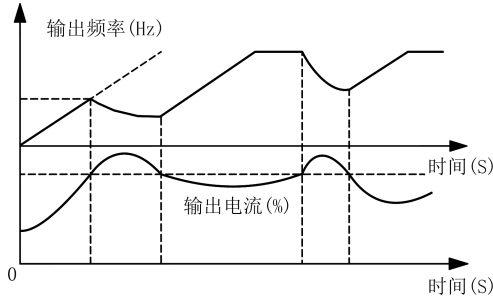
图 7- 25 电流限幅动作过程
