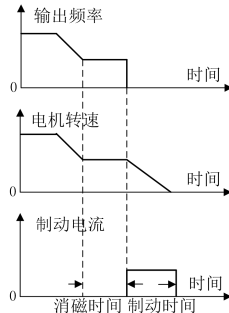
图 7- 18 停车直流制动过程
