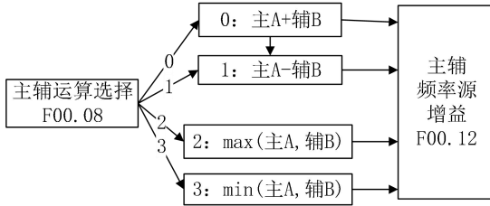
图 1- 4 主辅运算给定示意图
