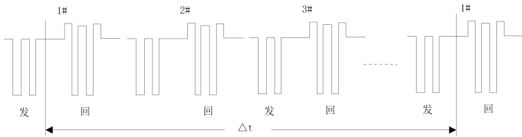
图 4- 24485 网络链路数据示意图
