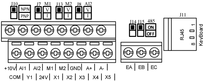
图 3- 11 控制回路端子排列
