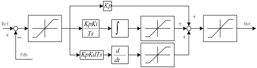
图 7-27 过程 PID 框图描述
