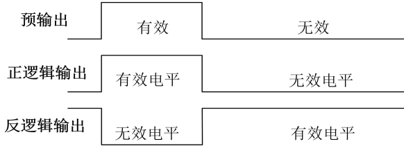
图 7- 14 数字输出端子正反逻辑输出示意图
