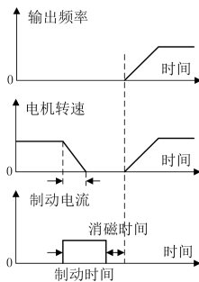
图 7- 17 启动直流制动过程
