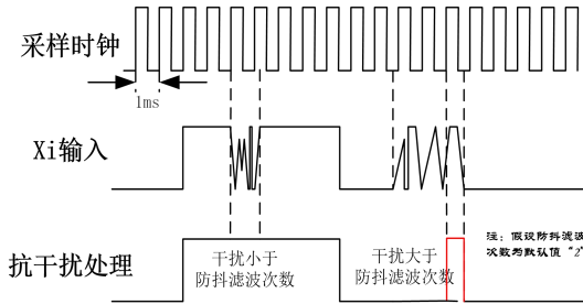
图 7- 13 端子滤波采样示意图
