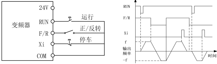
(c) F00.03=3 三线控制接线示意图 (d) F04.19=0, F00.03=3 正/反转运行逻辑 图 5-3 三线控制
