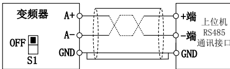
图 3-8 单台变频器通讯端子配线
