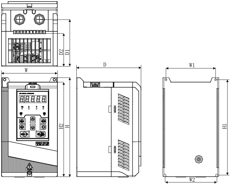
(b) 0.75kW~18kW 变频器外形
