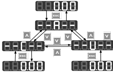
图 4-1 菜单模式选择操作流程图
