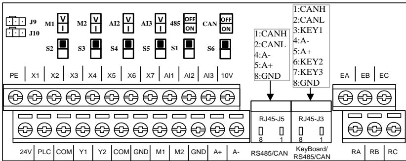
图 3-5 控制回路端子排列
