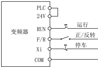
(c) F00.03=3 三线控制接线示意图 (d) F04.19=0, F00.03=3 正/反转运行逻辑 图 5-3 三线控制
