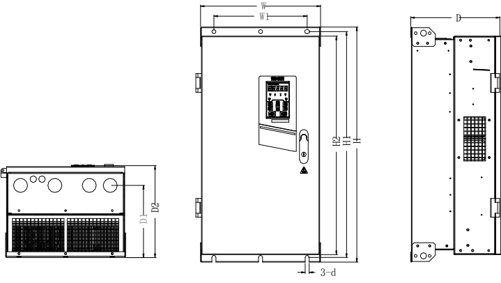
(d) 90kW~400kW 变频器外形
