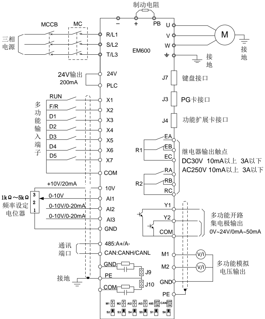
图 3-10 控制回路标准接线图
