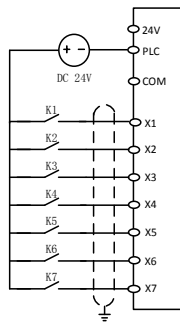
图 3-6 多功能输入端子接线图
