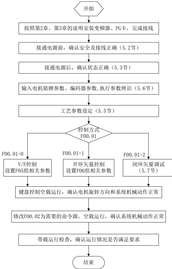
图 5-1 变频器闭环调试流程图
