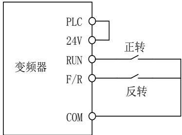
(c) F00.03=1 两线控制接线示意图
