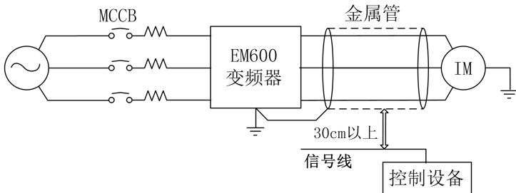
图 3- 9 感应干扰对策
