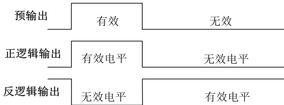
图 7- 15 数字输出端子正反逻辑输出示意图
