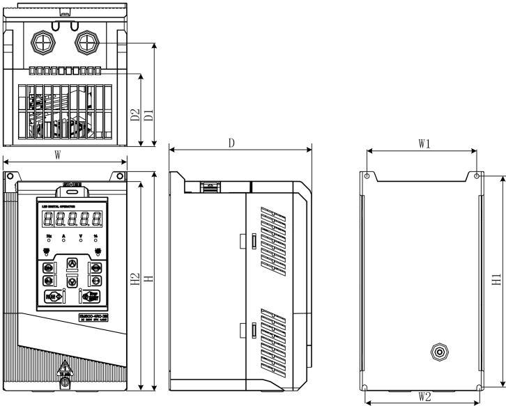
(b) 0.75kW~18kW 变频器外形
