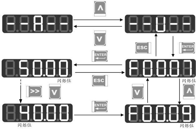
图 4- 6 自定义模式下功能代码的修改
