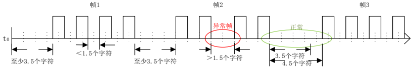
图 12-3 数据帧正误示意图
