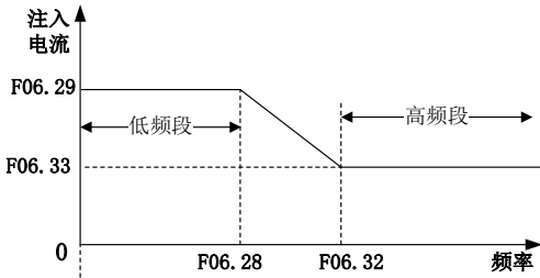
图 7-23 高频注入图示
