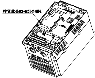
图附 6 I/O 扩展卡安装示意图
