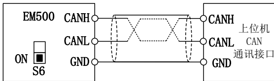
图 3-22 单台变频器 CANSinec 通讯配线
