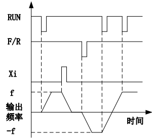
(a) F00.03=2 三线控制接线示意图 (b) F04.19=0, F00.03=2 正/反转运行逻辑
