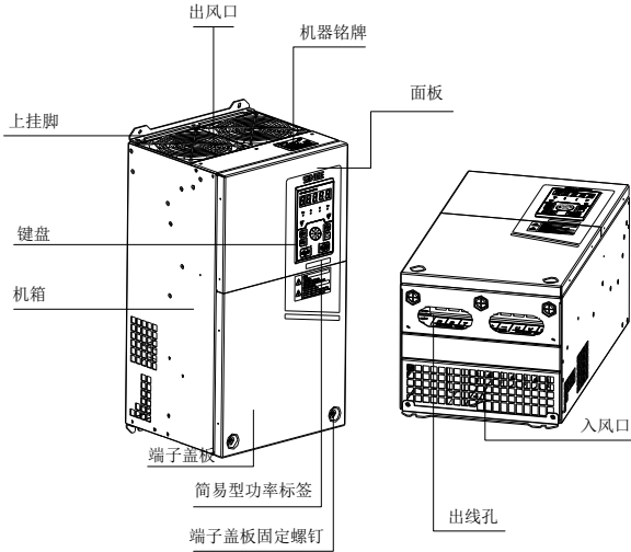
图 1-8 EM500 系列 30kW 变频器部件说明
