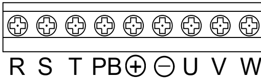
b) 11~18.5kW 各规格主回路端子
