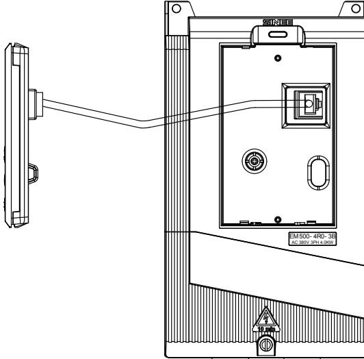
图 3-25 键盘延长线配线方式
