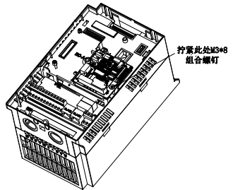
图附 4 DeviceNet 扩展卡安装示意图
