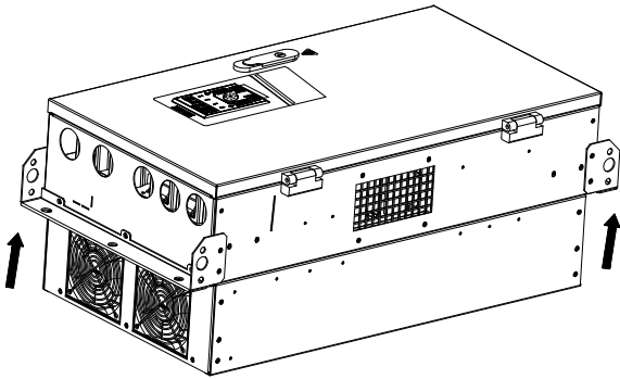
图 2-6 安装上下挂脚图示
