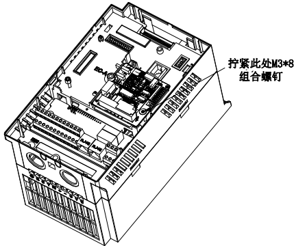
图附 2 I/O 扩展卡 3 安装示意图
