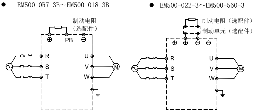
图 3-4 主回路标准接线
