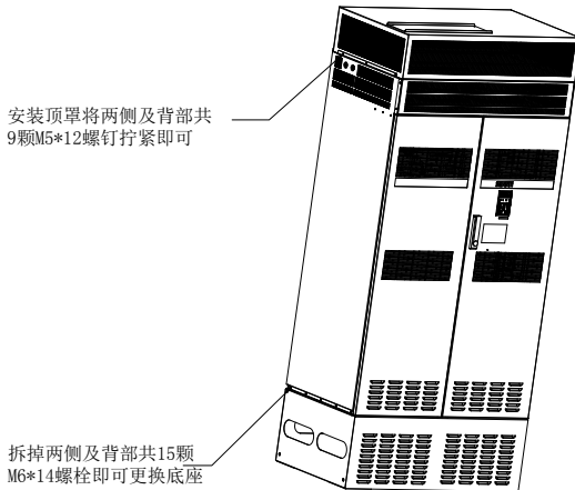
图 11-6 450~560kW 底座及頂罩安裝示意图
