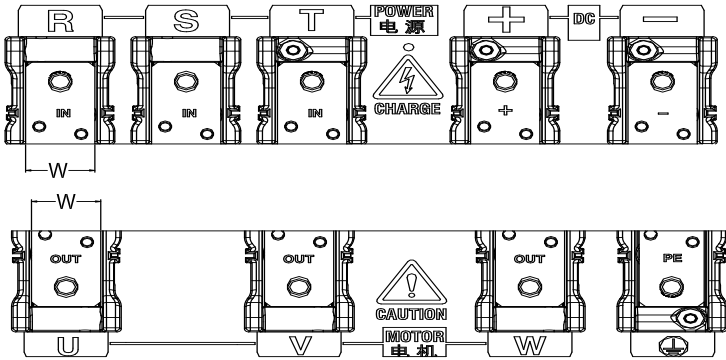
e) 90kW-200kW 规格主回路端子
