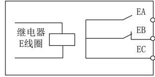
图 7-13 继电器触点
