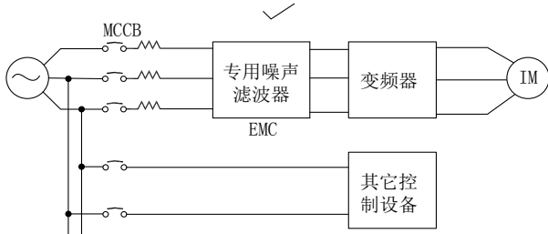
图 3-6 噪声滤波器的正确安装
