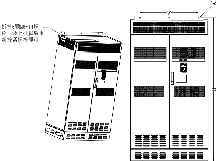
图 11-7 上挂脚安装示意图
