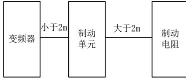
图 11-1 导线的长度
