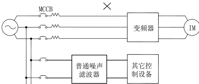
图 3-7 噪声滤波器的错误安装
