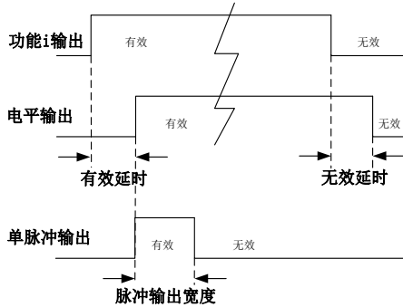
图 7-16 数字输出端子电平和单脉冲输出示意图
