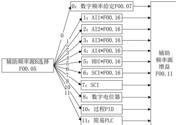
图 1-3 辅助频率源 B 给定示意图
