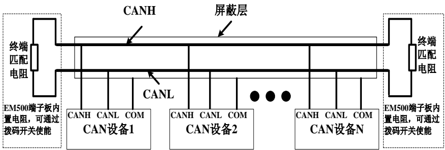
图 13-1 CAN 总线拓扑结构示意图
