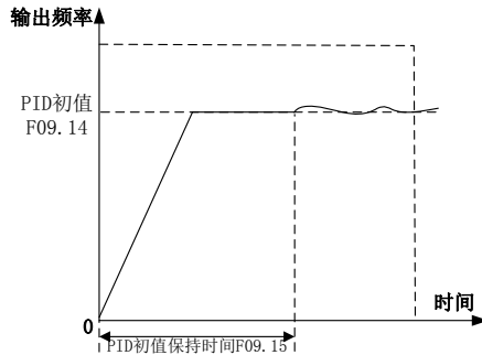
图 7-29 PID 初值输出示意图
