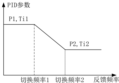
图 7-22PI 参数示意图
