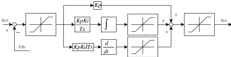
图 7-27 过程 PID 框图描述
