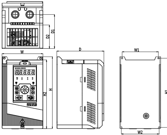
(b) 0.75kW~18kW 变频器外形
