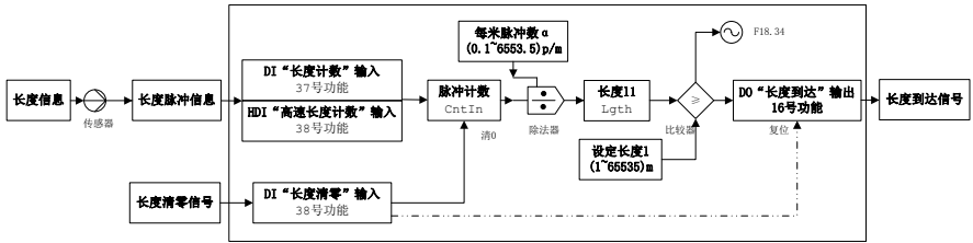
图 7-40 定长计数功能框图描述
