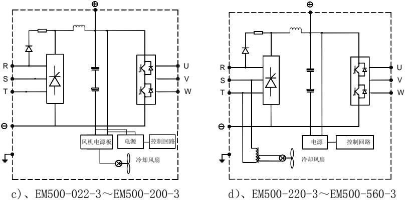
图 3-3 变频器内部主回路
