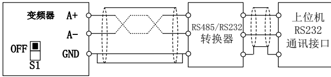
图 3-21 通讯端子配线
