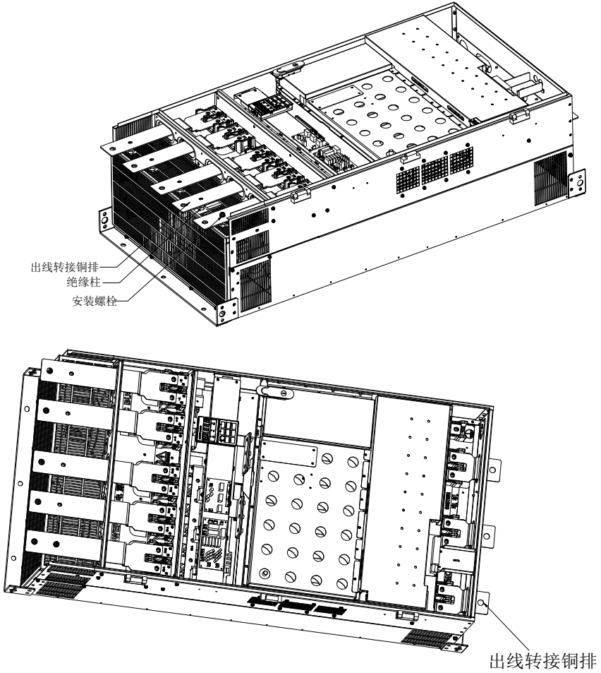
图 11-8 进出线转接铜排安装图示
