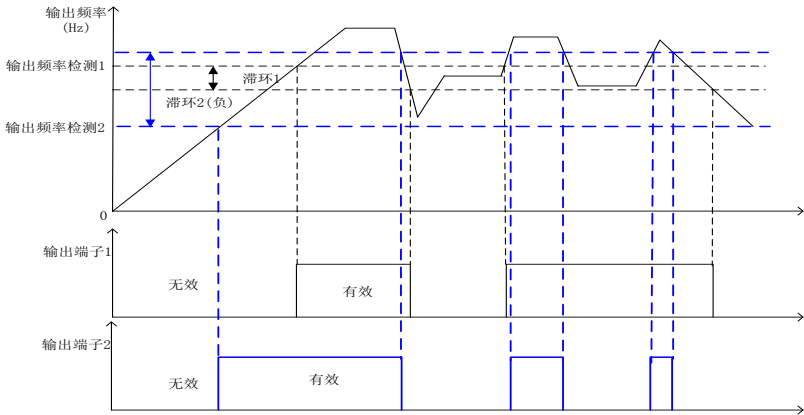
图 7-37 FDT 检测示意图
