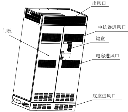
图 1-9 EM500 系列 450kW 变频器部件说明
