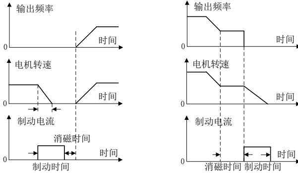
图 7-18 启动直流制动过程 图 7-19 停车直流制动过程
