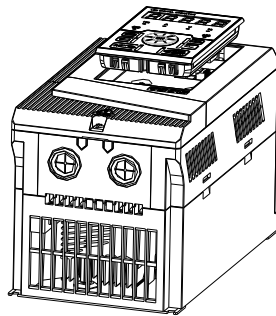
图 2-4 键盘安装图示
