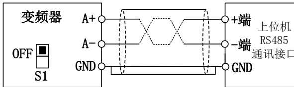
图 3-19 单台变频器通讯端子配线
