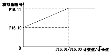
图 7-44 计数和计长模拟输出示意图
