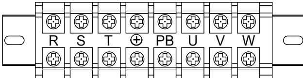
d) 45~75kW 各规格主回路端子（无内置制动单元的 PB 为 \ominus ）
