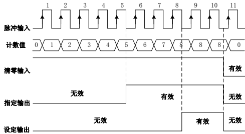
图 7-43 计数示例描述
