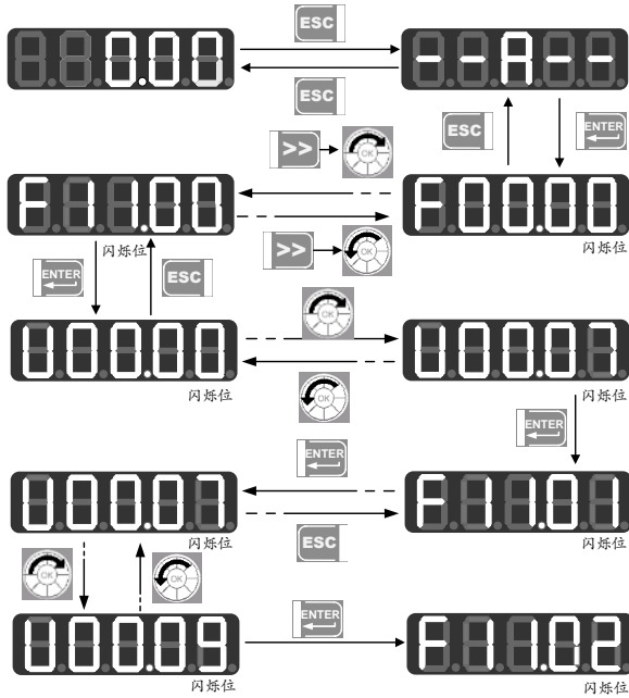
图 4-5 用户自定义模式设置示例
