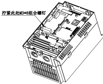
图附 7 I/O 扩展卡安装示意图
