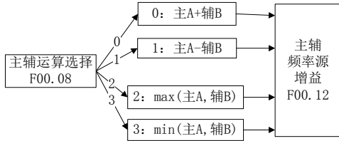
图 1-4 主辅运算给定示意图
