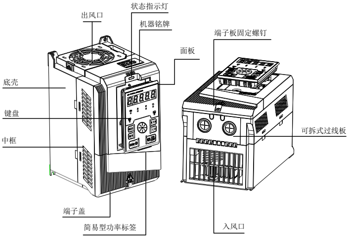
图 1-7 EM500 系列 4kW 变频器部件说明
