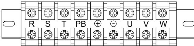
c) 22~37kW 各规格主回路端子
