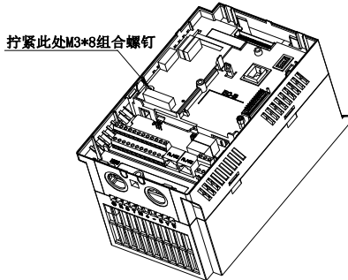
图附 5 I/O 扩展卡安装示意图
