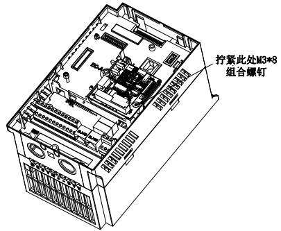
图附 3 CANopen 扩展卡安装示意图
