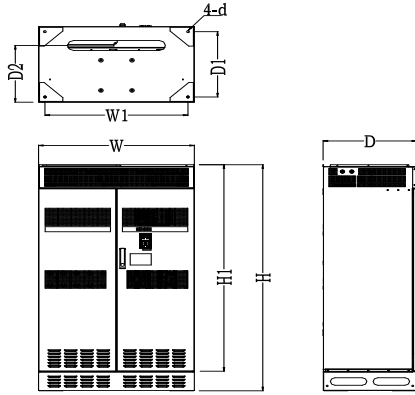
(e) 450~560kW 变频器外形
