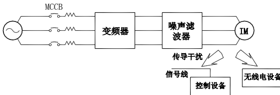
图 3-8 输出侧安装噪声滤波器
