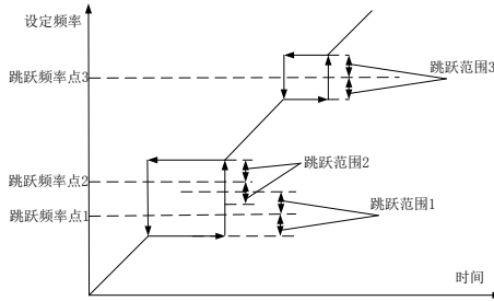
图 7-35 跳频示意图
