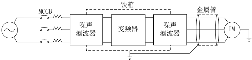
图 3-10 射频干扰对策
