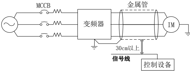
图 3-9 感应干扰对策
