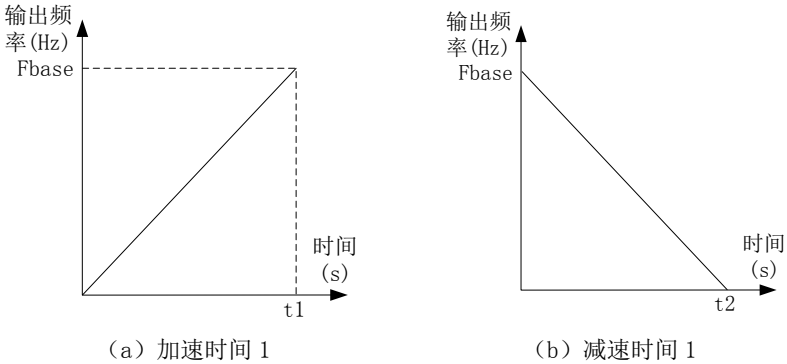
图 7-4 加减速时间
