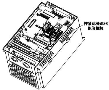
图附 1 IO 扩展卡安装示意图
