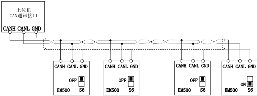
图 3-23 多台变频器 CANSinee 通讯配线
