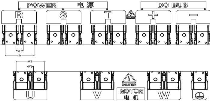
f) 220kW-400kW 规格主回路端子
